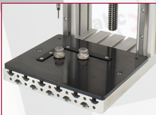
Tyypikilpi teline rajoittimilla (optio)
